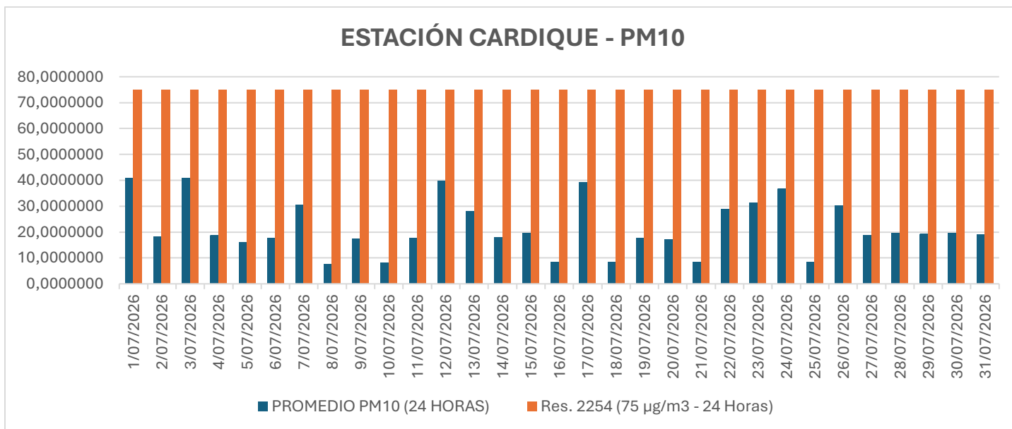
Gráfico 2. Concentración promedio de PM10 EST. CARDIQUE
