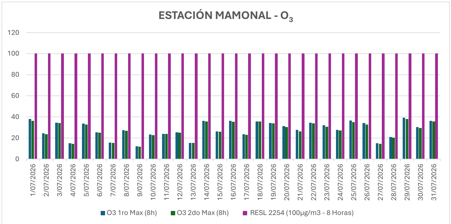
Gráfico 5. Concentración promedio de O 3 EST. MAMONAL
