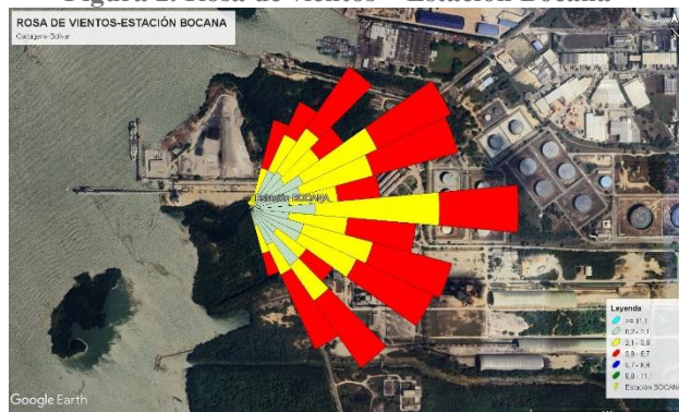
Figura 2. Rosa de vientos – Estación Bocana
