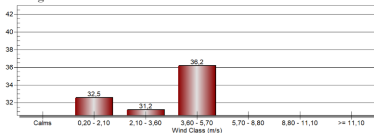
Figura 7. Distribución de frecuencia de vientos - Mamonal
