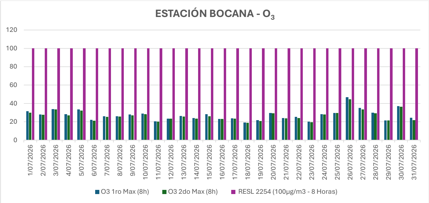
Gráfico 3. Concentración promedio de O 3 EST. BOCANA
