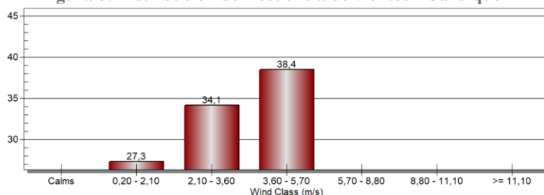
Figura 5. Distribución de frecuencia de vientos - Cardique
