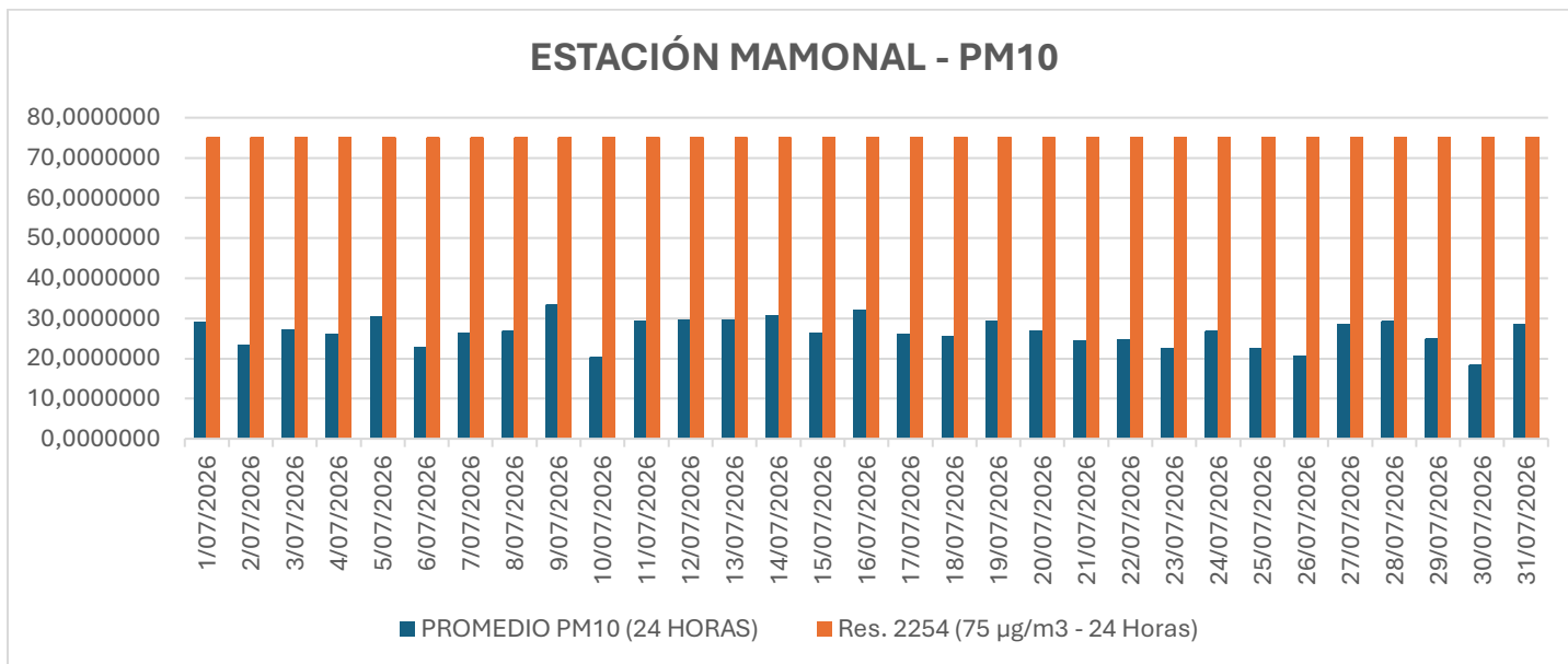
Gráfico 1. Concentración promedio de PM10 EST. MAMONAL
