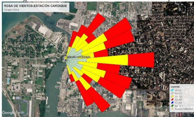
Figura 4. Rosa de vientos – Estación Cardique
