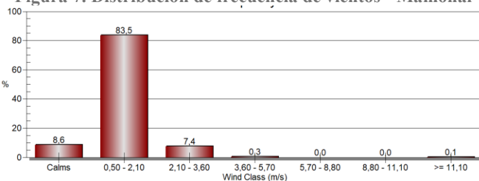
Figura 7. Distribución de frecuencia de vientos - Mamonal
