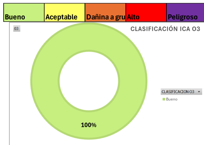
Gráfico 9. Índice de Calidad del Aire O 3 MAMONAL
