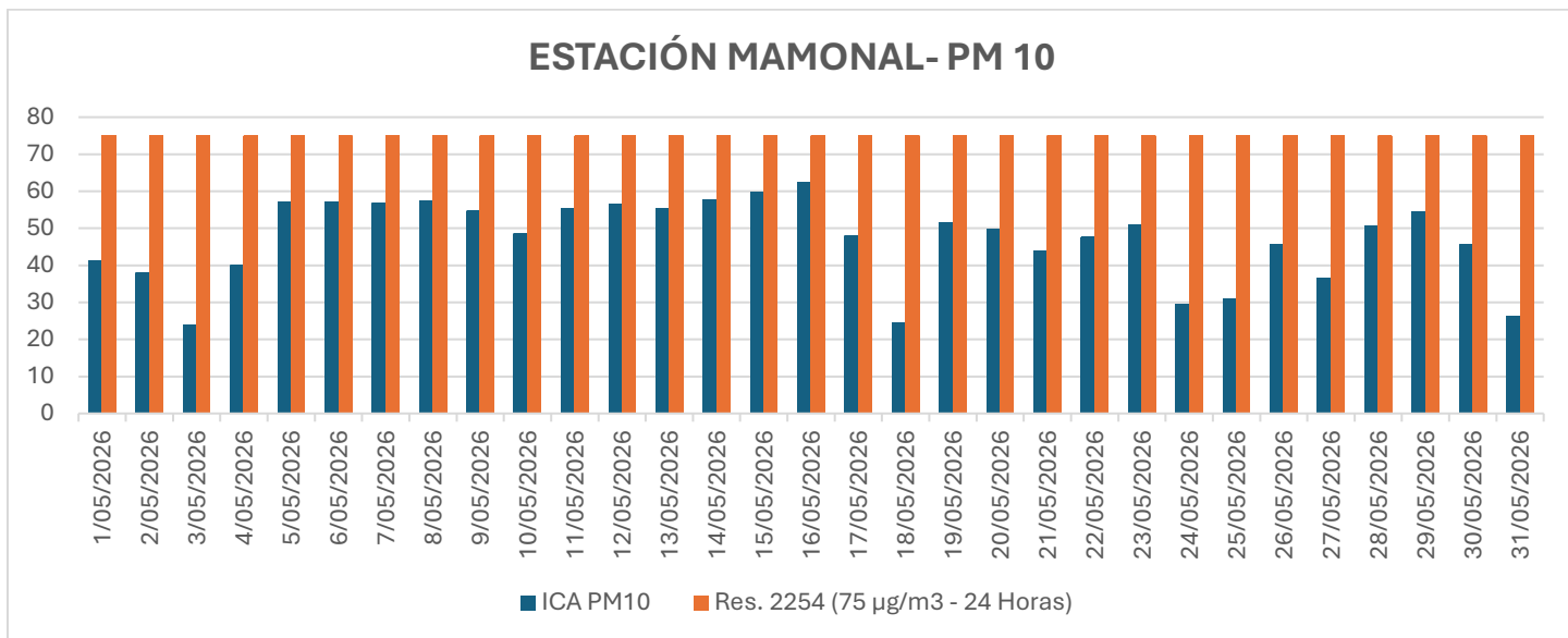
Gráfico 1. Concentración promedio de PM10 EST. MAMONAL
