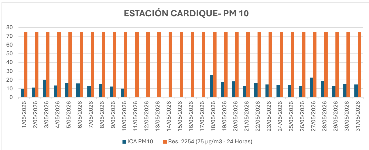
Gráfico 2. Concentración promedio de PM10 EST. CARDIQUE
