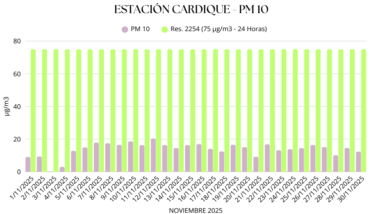
Gráfico 2. Concentración promedio de PM10 EST. CARDIQUE
