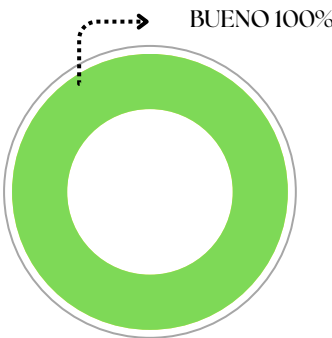
Gráfico 9. Índice de Calidad del Aire O3 MAMONAL.
