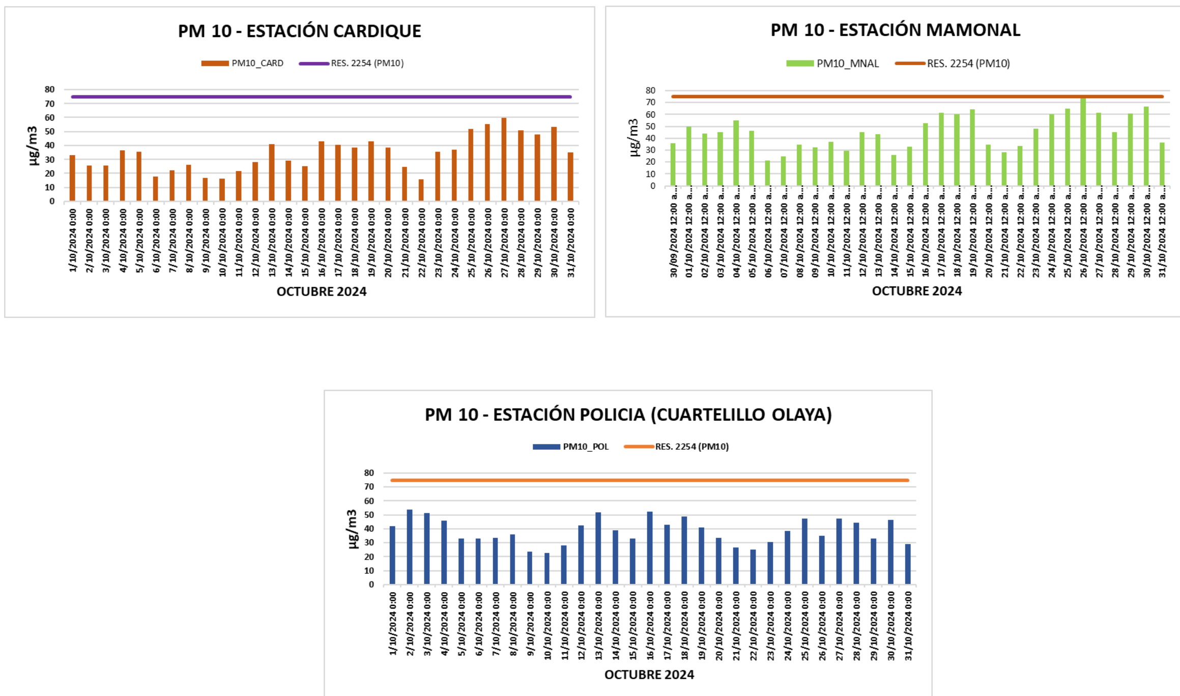
Gráfica 1. Concentraciones promedio mensuales de PM10 por estación de monitoreo – OCTUBRE.
