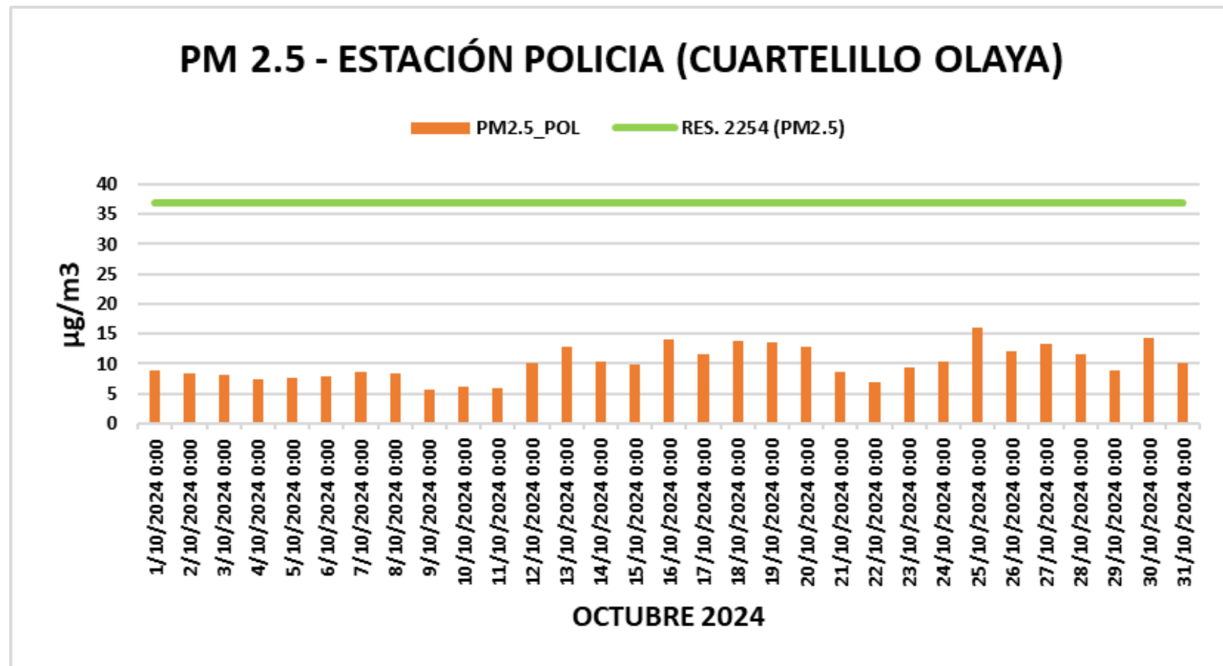
Gráfica 2. Concentraciones promedio mensuales de PM2.5 estación de policía (Cuartelillo de Olaya) – OCTUBRE.
