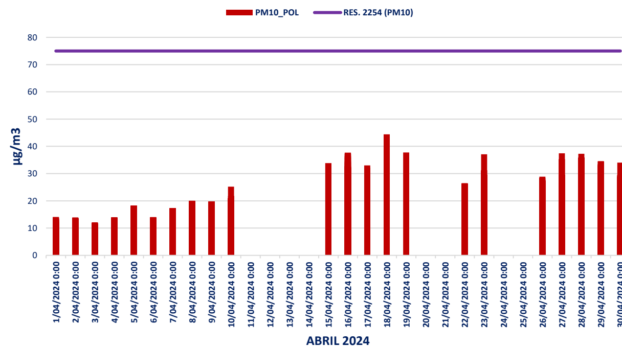
PM 10 - ESTACIÓN POLICIA (CUARTELILLO OLAYA)
