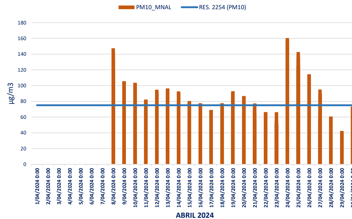
PM 10 - ESTACIÓN MAMONAL
