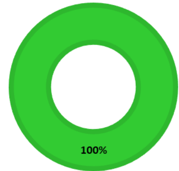
ICA PM 2.5_EST. POLICIA (CUARTELILLO OLAYA) ABRIL
