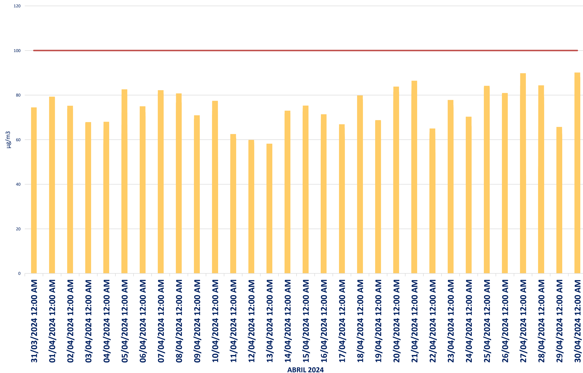
Gráfica 3. . Concentraciones de ozono- 8 horas
