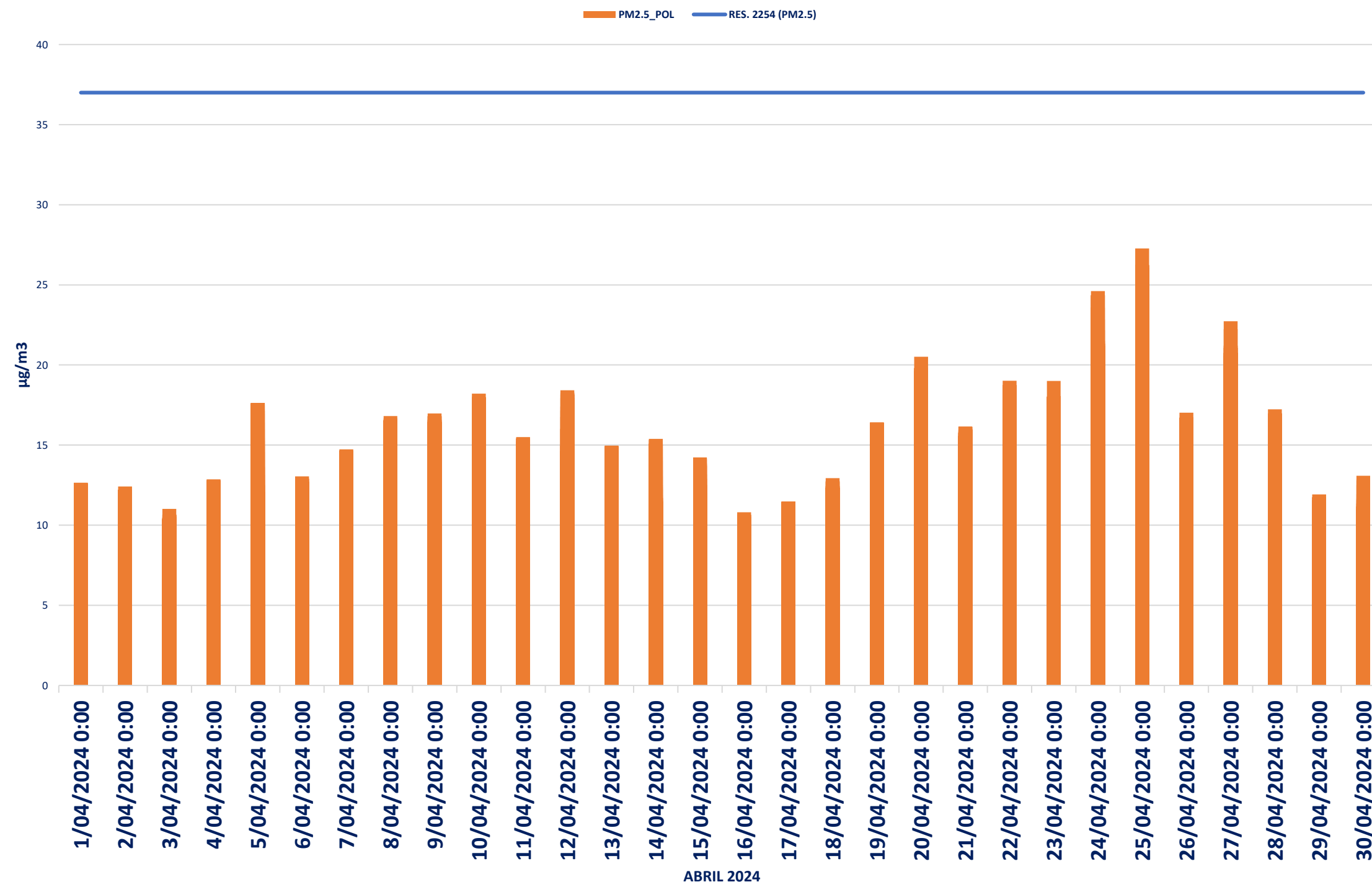
PM 2.5 - ESTACIÓN POLICIA (CUARTELILLO OLAYA)
