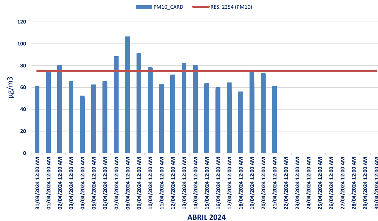
PM 10 - ESTACIÓN CARDIQUE.
